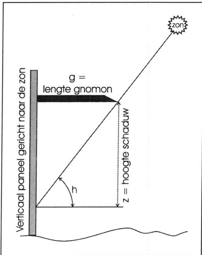
Figuur 2: aanduiding van de uurpunten op een verticale datumlijn. De gnomon moet altijd wijzen in de richting van de zon.
